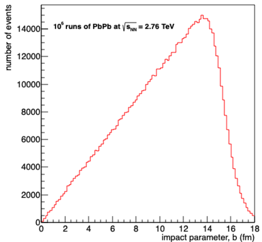
FIG. 7. Histogram of impact parameter values.
